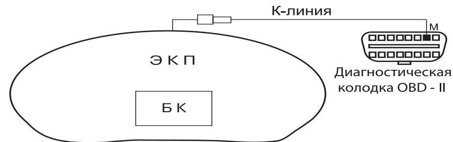
Рис. 1 Подключение БК
