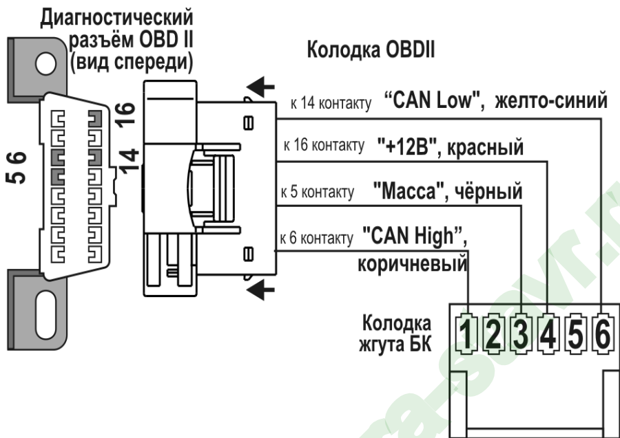
Рис.2 Схема подключения БК "ШТАТ GRANTA - X1"
