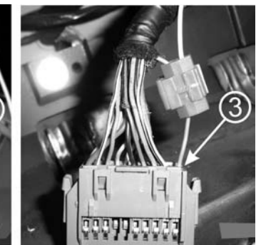
рис.12 Подключения проводов к колодкам комбинации приборов а/м Hyundai Getz
