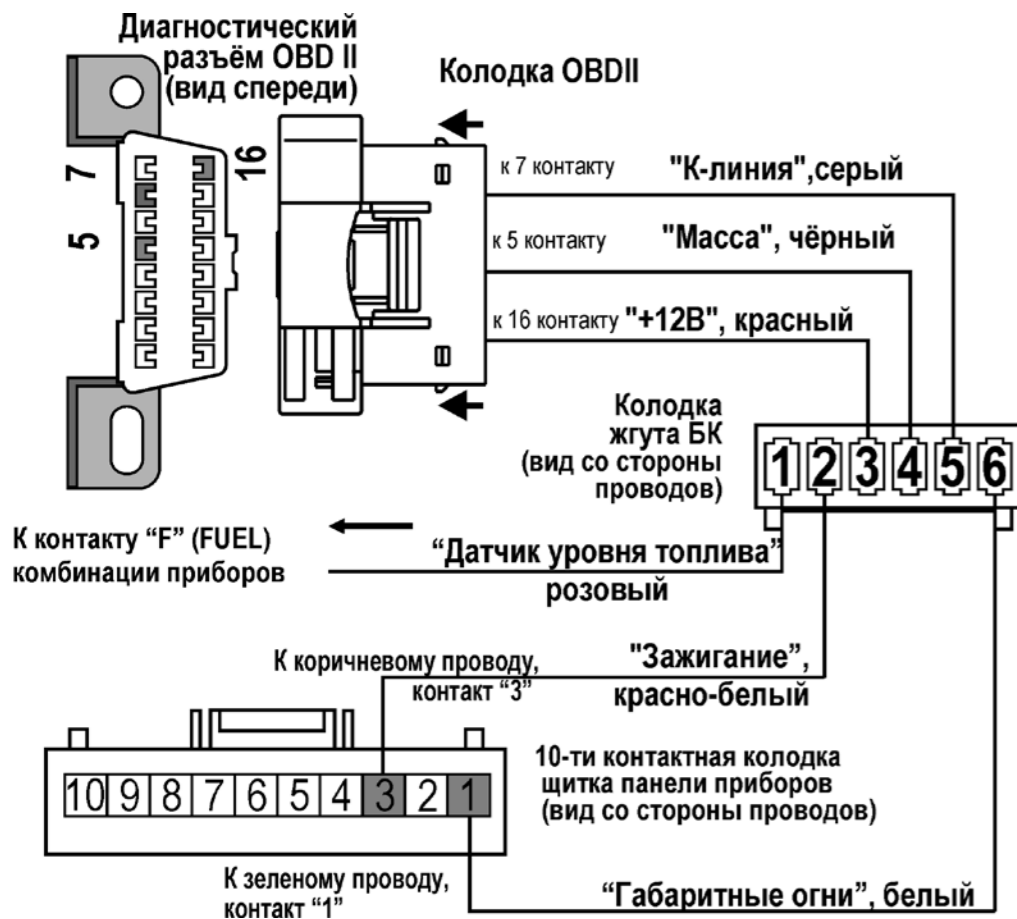
рис.8 Схема подключения к а/м Hyundai Accent
