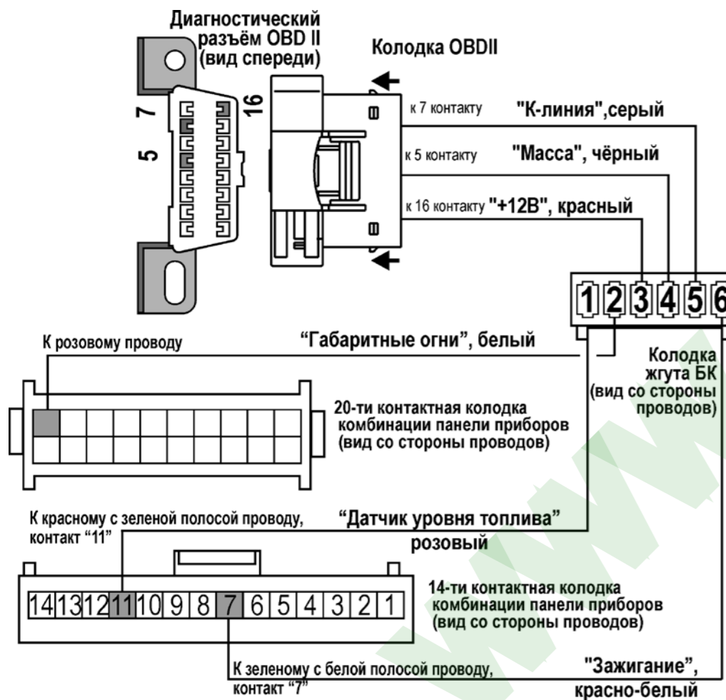
рис.9 Схема подключения к а/м Hyundai Getz
