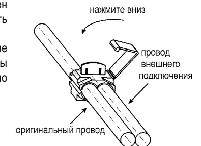
рис.13 Соединение проводов через зажим
