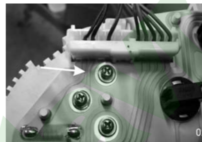
рис.10 Подключения ДУТ на а/м Hyundai Accent
