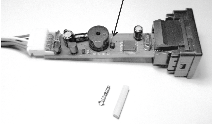
Порядок подключения вывода «Зажигание / ДУТ»
