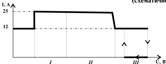
Вольт-Амперная характеристика работы НПП Орион-410 (схематично)
