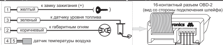
7-контактный разъем переходника
